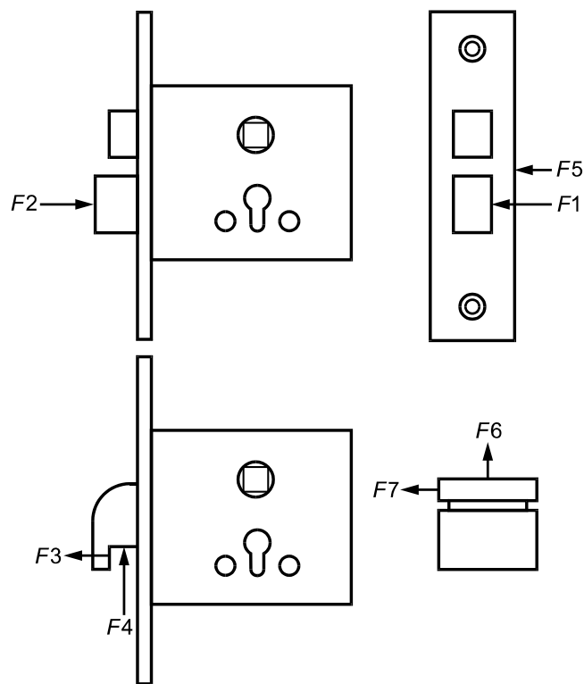
Рисунок 1 — Точки приложения сил, воздействующих на механизм замка
